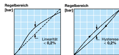
Linearität
